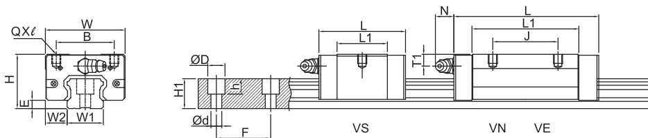
SRS-V 低组装系列规格尺寸表
