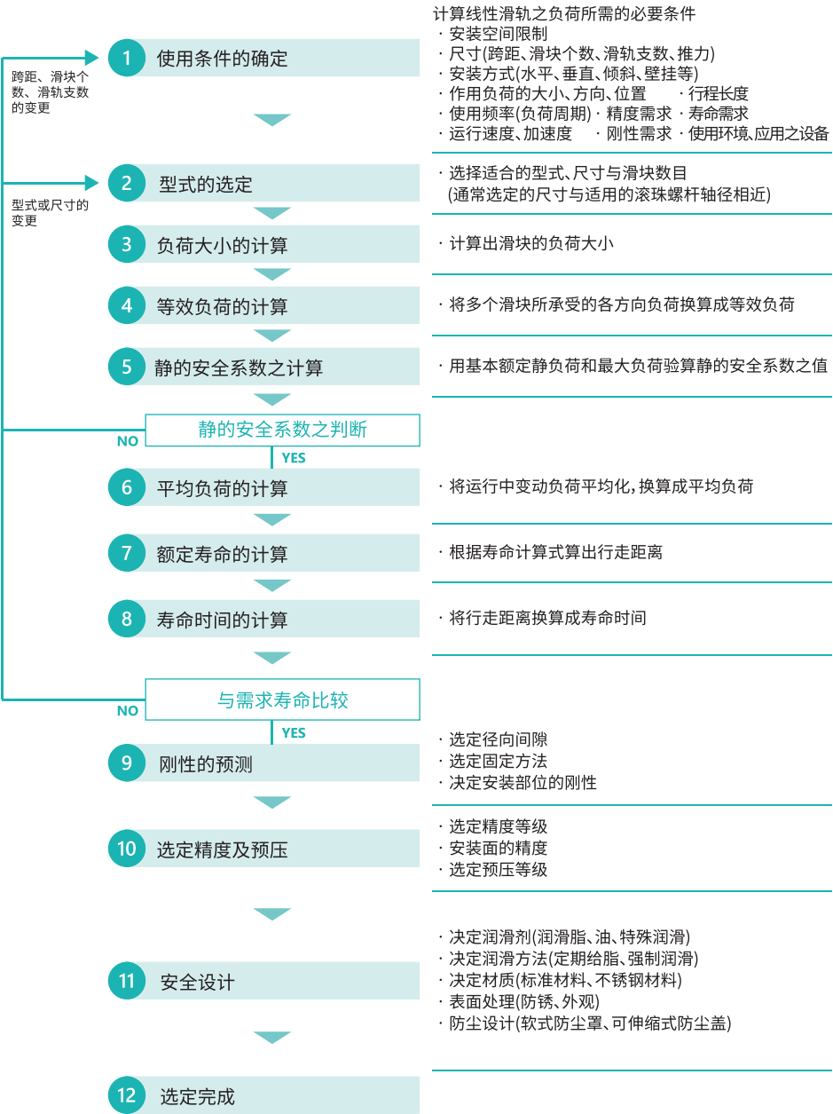
■ 1-2-1 线性滑轨的选定步骤流程图
