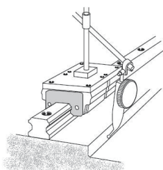
图 1.11.19 利用假基准面的方法
