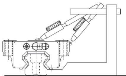
图 1.9.1 行走平行度
