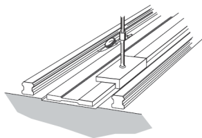
图 1.11.14 用直线块规的方法
