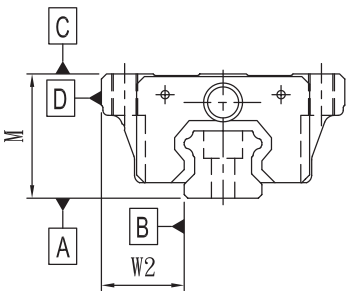
图 2.5.1 精度标准
