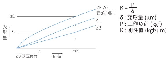
图 1.10.2 刚性数据
