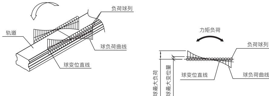
图 1.6.1 力矩作用时球的负荷
