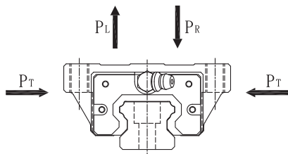
图 1.6.3 滑轨的负荷方向、力矩方向
