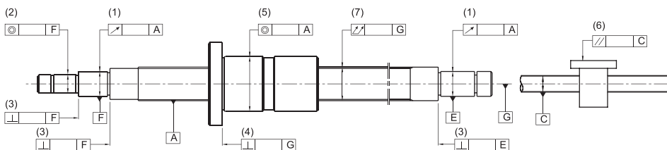
图 1.3.1 滚珠螺杆安装部位的精度 (ISO 3408)
