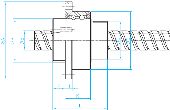
RFSY
