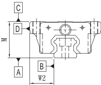
图 2.5.1 精度标准
