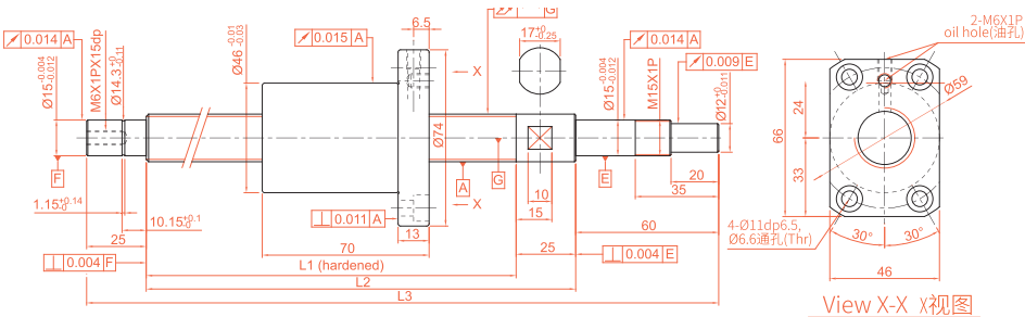
XSVR02020-00 精密研磨级系列规格尺寸表（研磨级轴端完成品）
