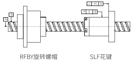
图 1.2.2 RBLY 系列
