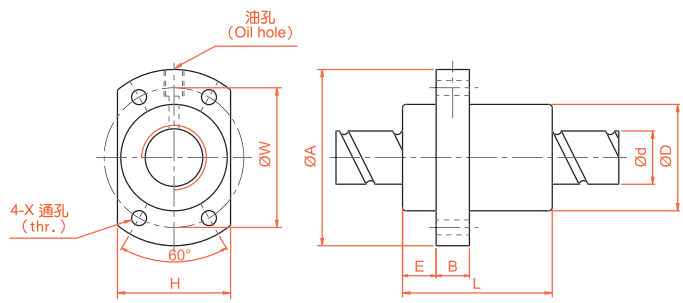
SFYA 转造级系列规格尺寸表
