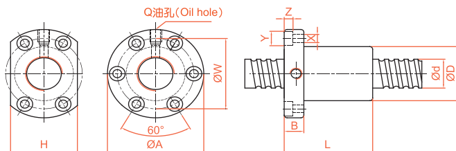
SFNI/SFI 转造级系列规格尺寸表
