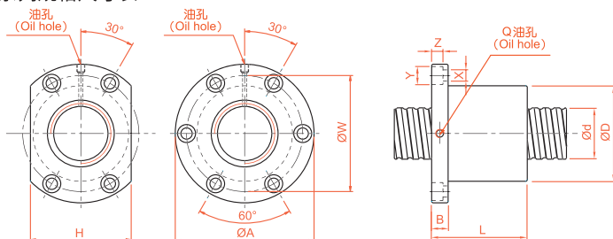
SFV 转造级系列规格尺寸表
