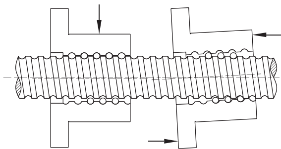
图 1.10.3 偏荷重
