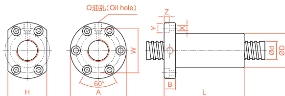
OFI 精密研磨级系列规格尺寸表
