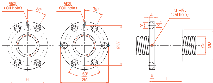
SFV 精密研磨级系列规格尺寸表
