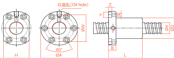
SFNI/SFI 精密研磨级系列规格尺寸表
