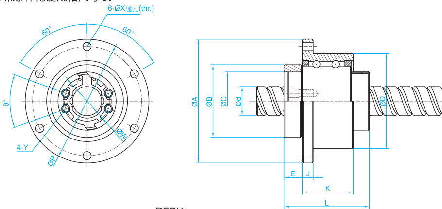
RBBY 精密滚珠螺杆花键规格尺寸表
