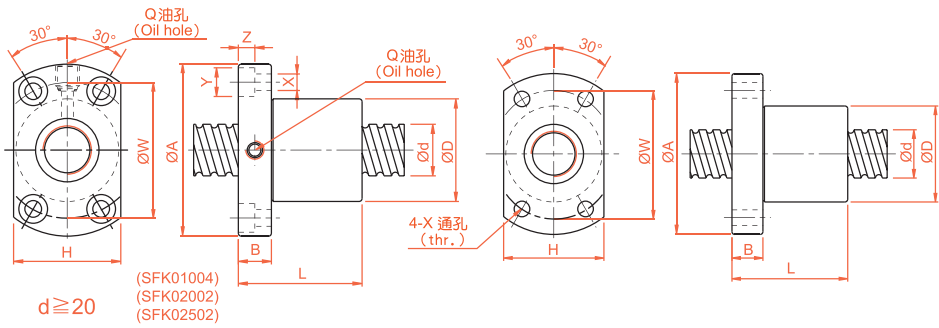
SFK 转造级系列规格尺寸表
