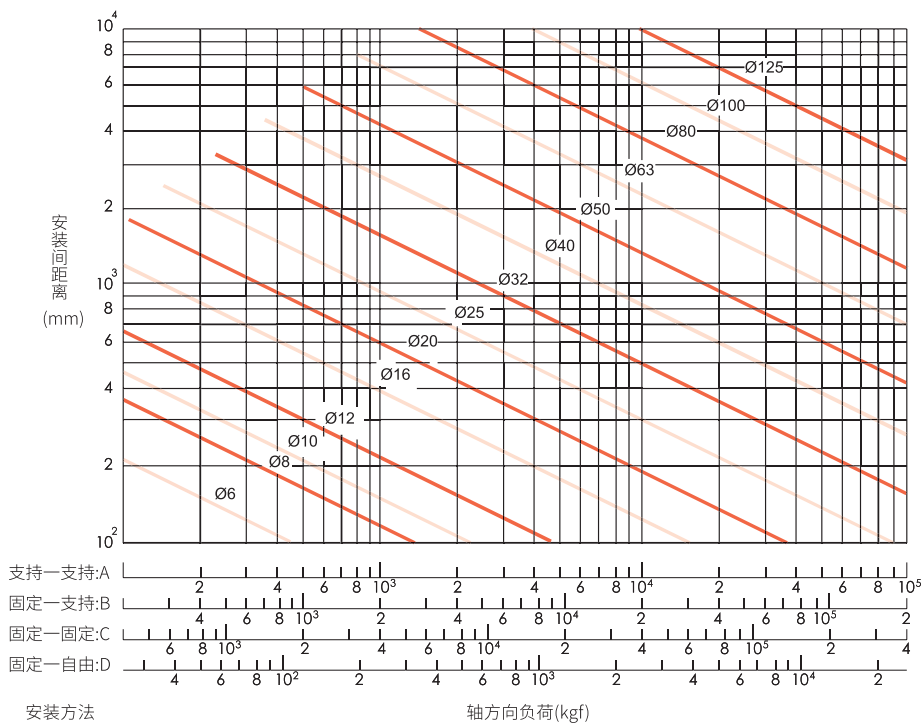
图 1.4.16 挫屈之容许压缩负荷
