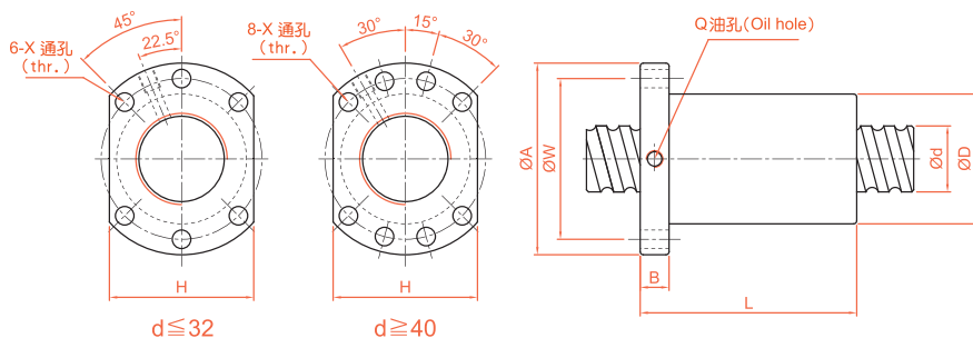
OFU (DIN 69051 FORM B) 精密研磨级系列规格尺寸表
