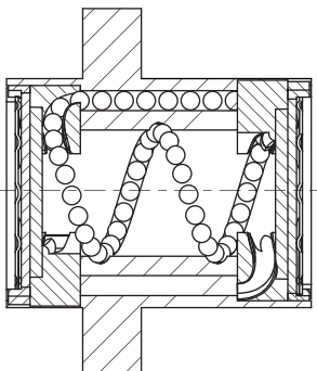
图 1.6.4 Y, YA, A, J 型螺帽图
