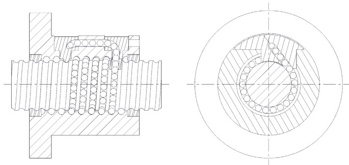
图 1.6.3 V 型螺帽图
