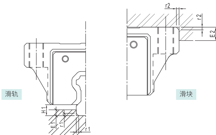
图 1.11.21
