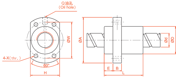
SFYA 精密研磨级系列规格尺寸表
