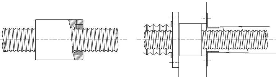
图 1.10.2 防尘机构
