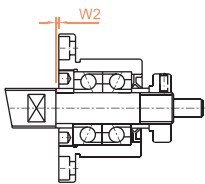
H2 型
