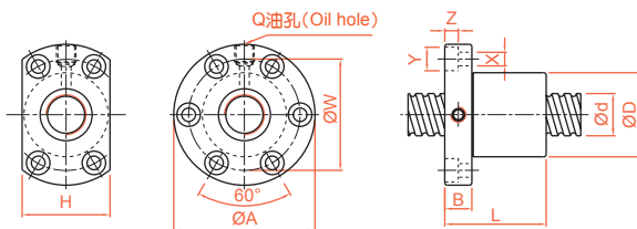
SFM 转造级系列规格尺寸表 (铣床专用)
