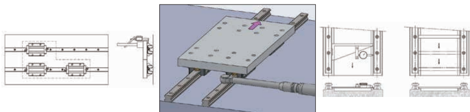
图 1.11.15 移动工作台的方法
