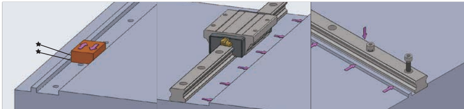
图 1.11.6 安装前的检查
