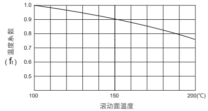
图 1.3.3 温度系数 (f t )
